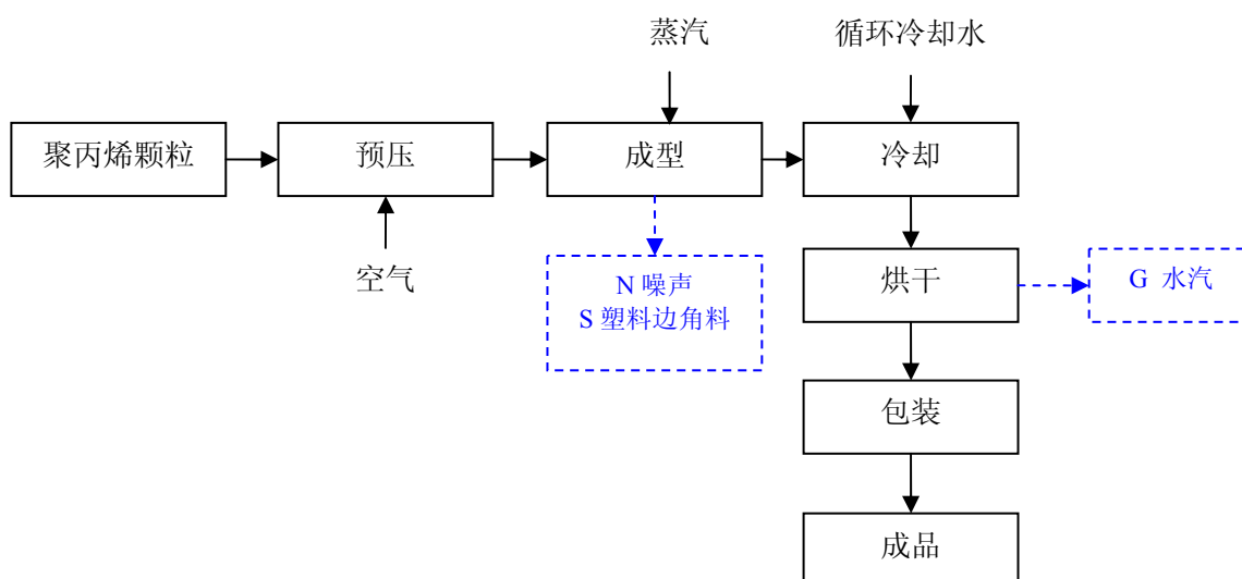
图 2-2 聚丙烯包装材料生产工艺图
