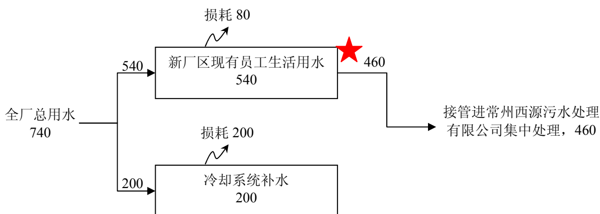
图 2-1 全厂水平衡图 单位：吨/年
